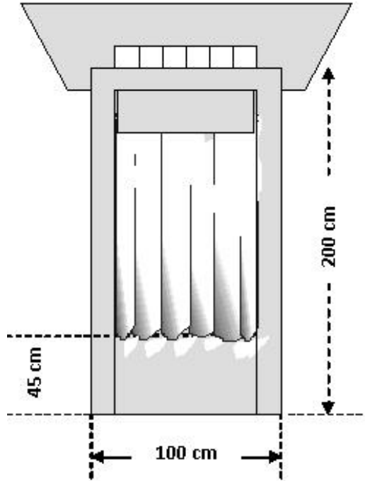
Tampak Depan
